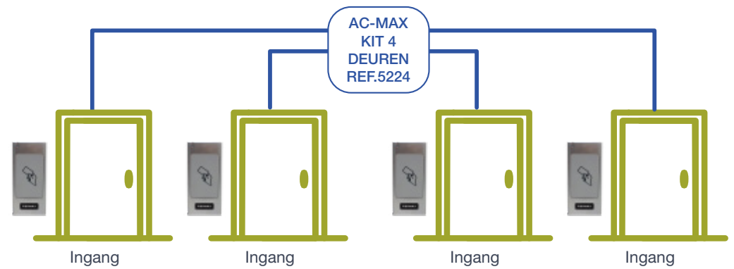
INSTALLATIE MET 4 DEUREN
