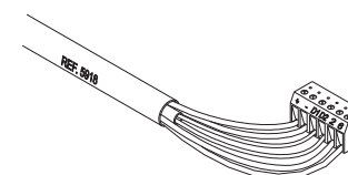
Dekoder-Bus Verdrahtung
