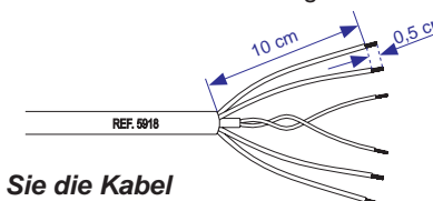
Dekoder-Bus Verdrahtung
