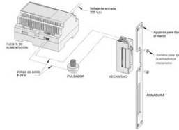
Esquema de instalación unifilar (imagen)
