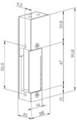
Imagen de cotas
